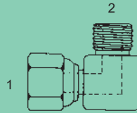
BPP-FJX-6501 - 90° (1) 37° Fem. Swivel (2) Male BPP
