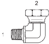
Y-1501-F-R - 90°
