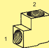
BIF-452 - 90° (1) Fem. Inv. Flare (2) Fem. Pipe
