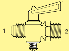
BV-204F - Str. (1) Male 45° Flare (2) Male Pipe
