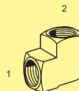
BP-5504 - 90°
