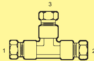
B-IE-84-LB - Tee (1) (2) (3) Tube
