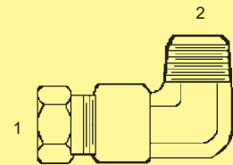
B-IE-89-LB - 90° (1) Tube (2) Fem. Pipe
