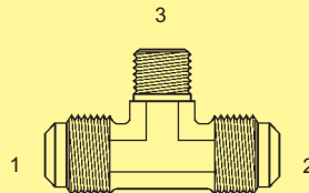
BF-2601-F - Tee
