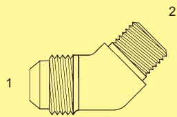
BF-2503 - 45°
